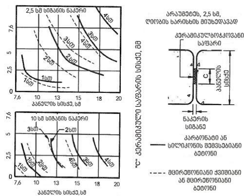
სურ. 722.2.1.3.1 კერამიკ-ბოჭკოს ზმულის დამცავი
